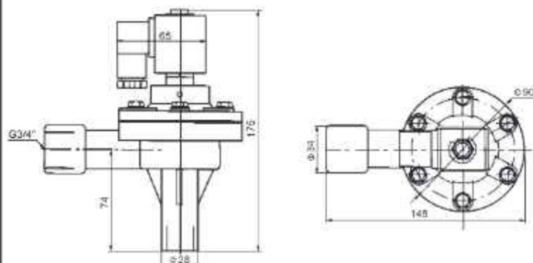
DMF-Z-20/25
